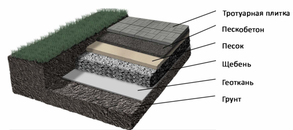
Поперечный профиль мощения тротуарной плиткой
